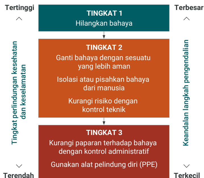
Gambar 1 Hirarki pengendalian
